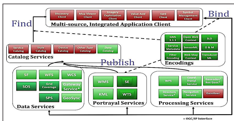
Figura 1. Framework de servicios web de estándares de Geoprocesamiento OGC. (OSGeoLive, 2012).
