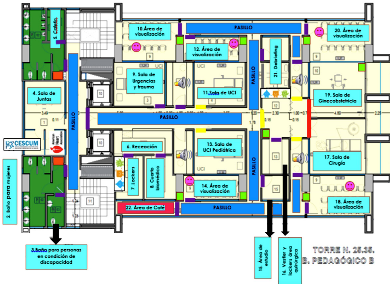
Figura 2. Planos arquitectónicos Hospital simulado Universidad de Manizales
